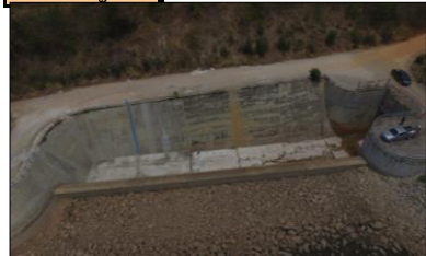
อาคารระบายน้ำล้น อ่างเก็บน้ำคลองโพธิ์
